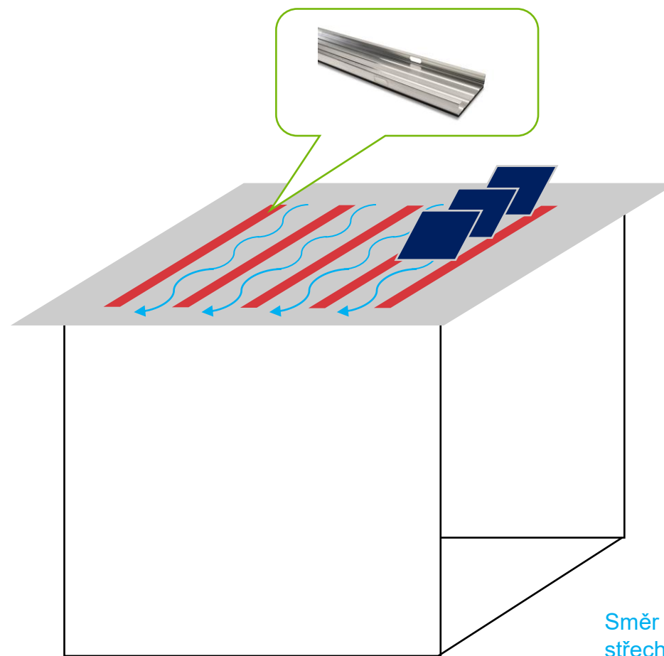
Základní žlab s ochranným pásem
